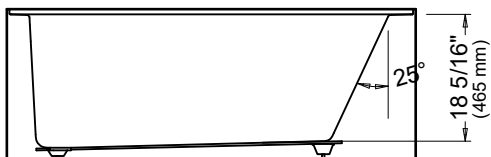
Vue arrière
